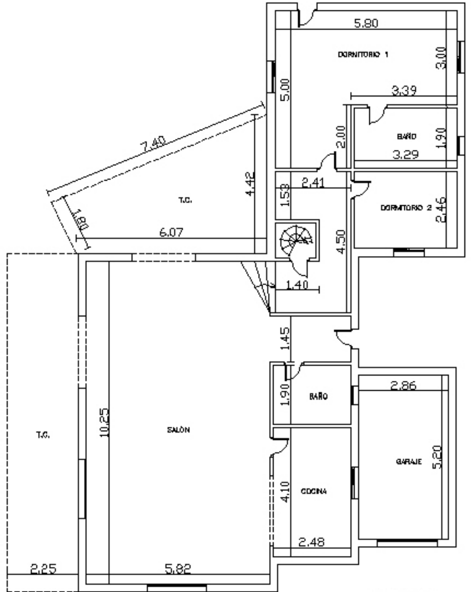
PLANTA BAJA VIVIENDA PRINCIPAL
